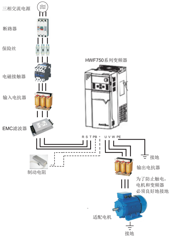
图2-1 HWF750系列系统构成
