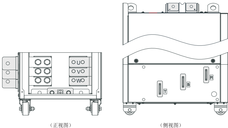
图3-5 HWF750T200G~HWF750T450G主回路端子分布图
