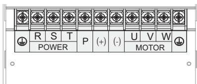
图3-4 HWF750T45G~HWF750T185G主回路端子分布图
