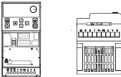
图3-3 HWF750T0.7G(B)~HWF750T37G(B)主回路端子分布图
