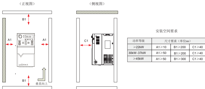
图3-1 单台机器 HWF750系列安装空间
