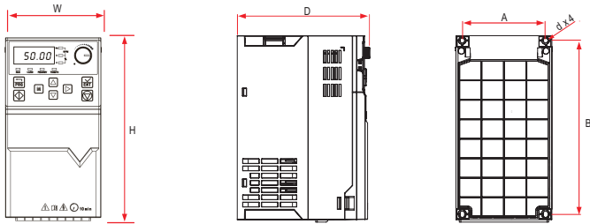
图8-3 HWF750T0.7GB-HWF750T185G外型尺寸及安装尺寸示意图
